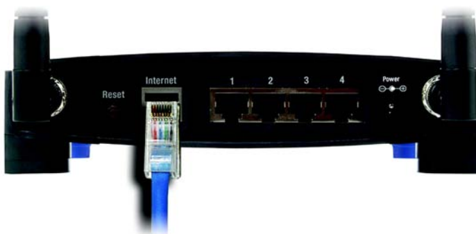
Afbeelding 4-1: Uw internetverbinding aansluiten
