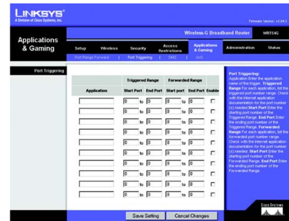
Figur 6-34: Fliken Applications and Gaming (Tillämpningar och spel) – Port Triggering (Portutlösning)
