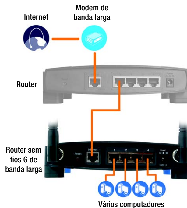
Figura 4-4: Diagrama para ligação a outro router
