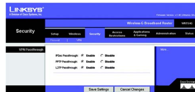
Figur 6-27: Fliken Security (Säkerhet) – VPN Passthrough (VPN-genomströmning)
