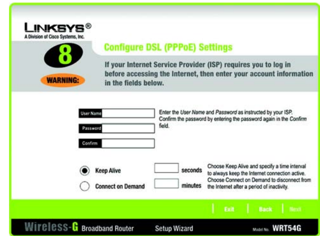
Figura 5-11: Pantalla Configure DSL (PPPoE) Settings (Configurar los parámetros de DSL, PPPoE) del asistente de configuración
