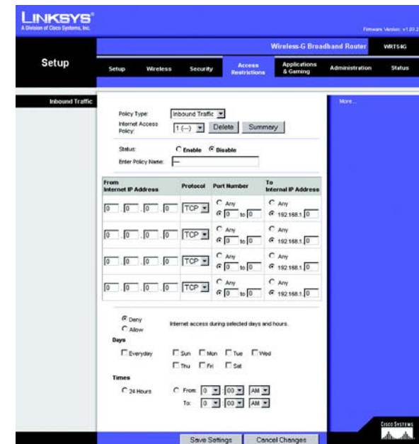
Figur 6-32: Fanen Access Restrictions - Inbound Traffic (Adgangsbeskrænsning - Indgående trafik)
