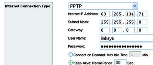
Abbildung 6-6: Verbindungstyp „PPTP“
