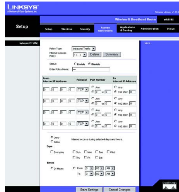
Afbeelding 6-32: Tabblad Access Restrictions (Toegangsbeperkingen) - Inbound Traffic (Inkomend verkeer)
