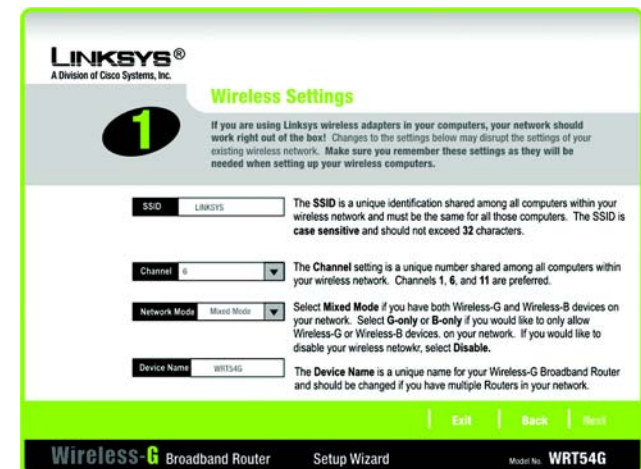
Abbildung 5-28: Setup-Assistent – Fenster Wireless Settings (Wireless-Einstellungen)
