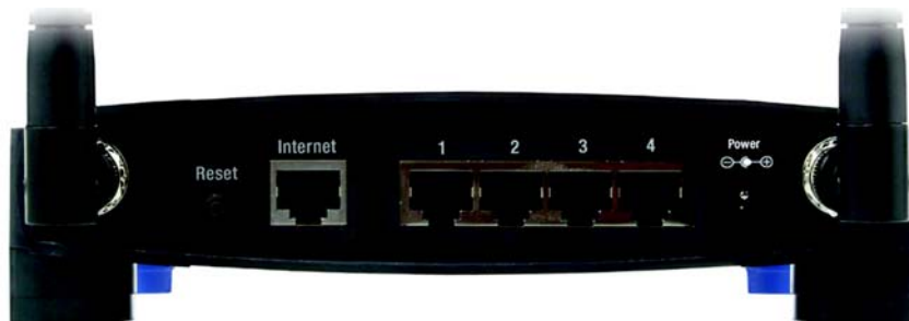
Figura 3-1: Panel posterior del ruteador
