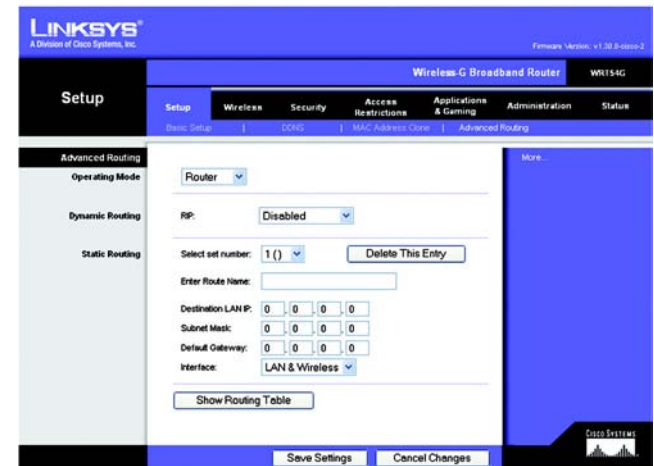
Abbeelding 6-15: Tabblad Setup (Instellingen) - Advanced Routing (Geavanceerde routing) (router)
