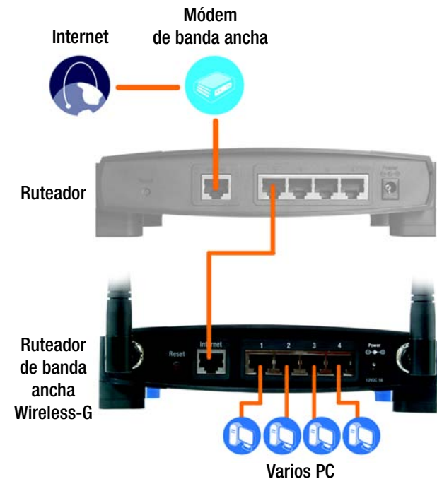
Figura 4-4: Diagrama para la conexión a otro ruteador
