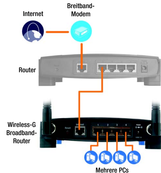
Abbildung 4-4: Beispiel für eine Verbindung mit einem anderen Router
