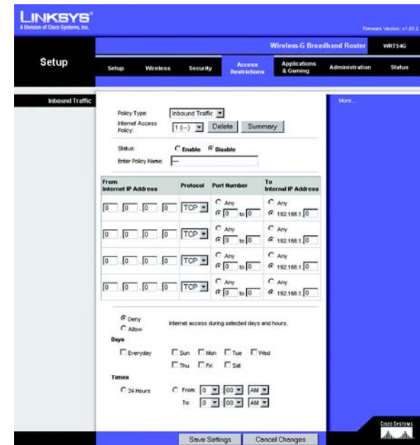
Abbildung 6-32: Registerkarte „Access Restrictions“ (Zugriffsbeschränkungen) – „Inbound Traffic“ (Eingehender Datenverkehr)
