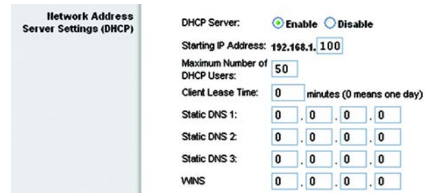
Figura 6-10: Network Address Server Settings (Definições do servidor de endereços de rede)
