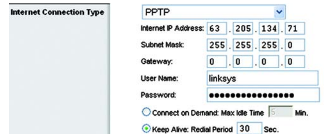
Figura 6-6: Tipo de conexión PPTP
