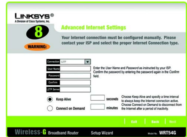
Figura 5-15: Ecrã Advanced Internet Settings - L2TP (Definições de Internet avançadas - L2TP) do assistente de configuração
