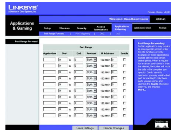
Figura 6-33: Scheda Applications and Gaming (Applicazioni e giochi) - Port Range Forward (Inoltro intervallo porte)
