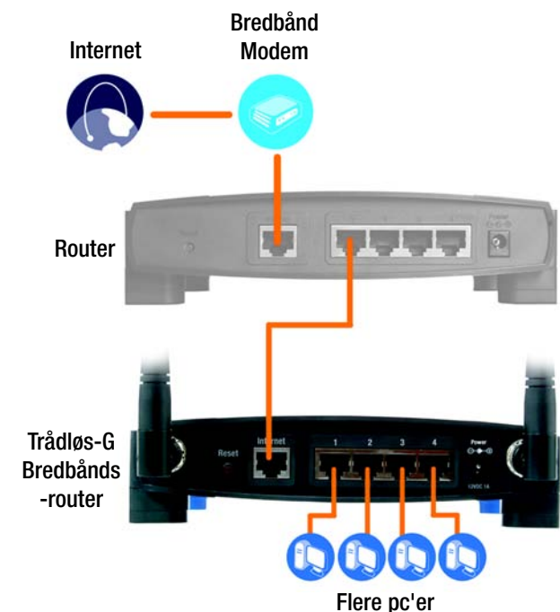
Figur 4-4: Diagram for tilslutning til en anden router
