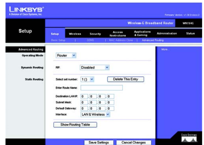
Figura 6-15: Scheda Setup (Configurazione) - Advanced Routing (Routing avanzato) (Router)
