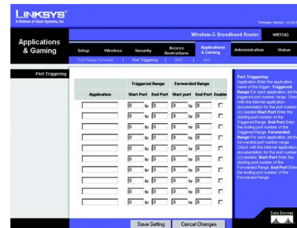
Figur 6-34: Fanen Applications & Gaming - Port Triggering (Programmer og spil - Aktivering af porte)
