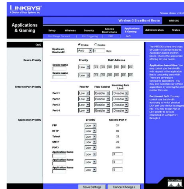
Abbildung 6-36: Registerkarte „Applications & Gaming“ (Anwendungen & Spiele) – „QoS“
