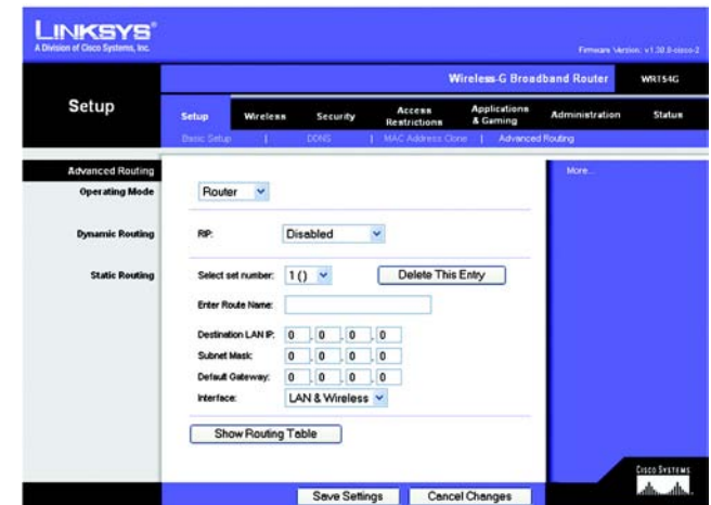
Abbildung 6-15: Registerkarte „Setup“ (Einrichtung) – „Advanced Routing (Router)“ (Erweitertes Routing (Router))
